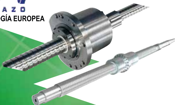
HUSILLOS DE BOLAS DE GRAN TAMAÑO
