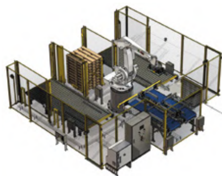
Sistemas de paletizado / Robot aplicador
