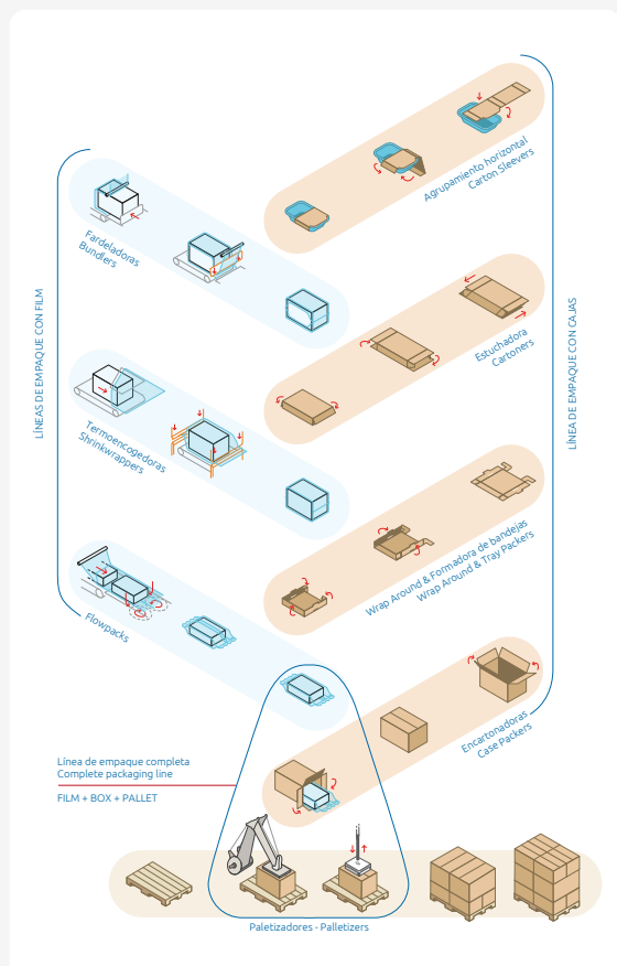
Encartonadoras automáticas y armadoras y cerradoras de cajas
