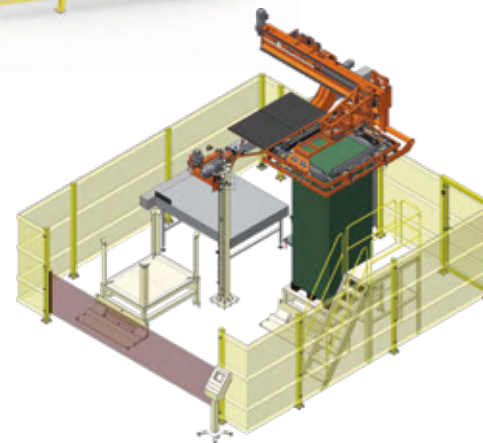
Sistemas convencionales de manipulación de paletizado y despaletizado
