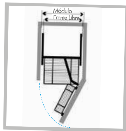
Apertura máxima: 90° Maximum door opening 90° Vista superior derecha - Abierta Right top view - Open
