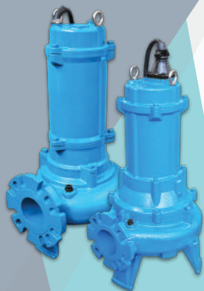
DESAGÜE Serie KTM 2 - 20 HP
