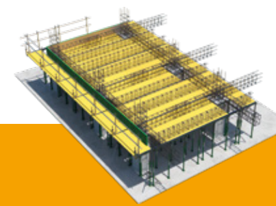
05 ENCOFRADO HORIZONTAL TRICAPA
