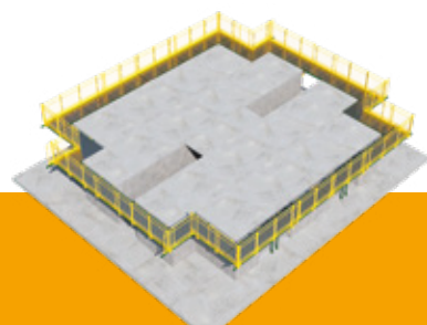
02 ANDAMIO TIPO CANASTA
